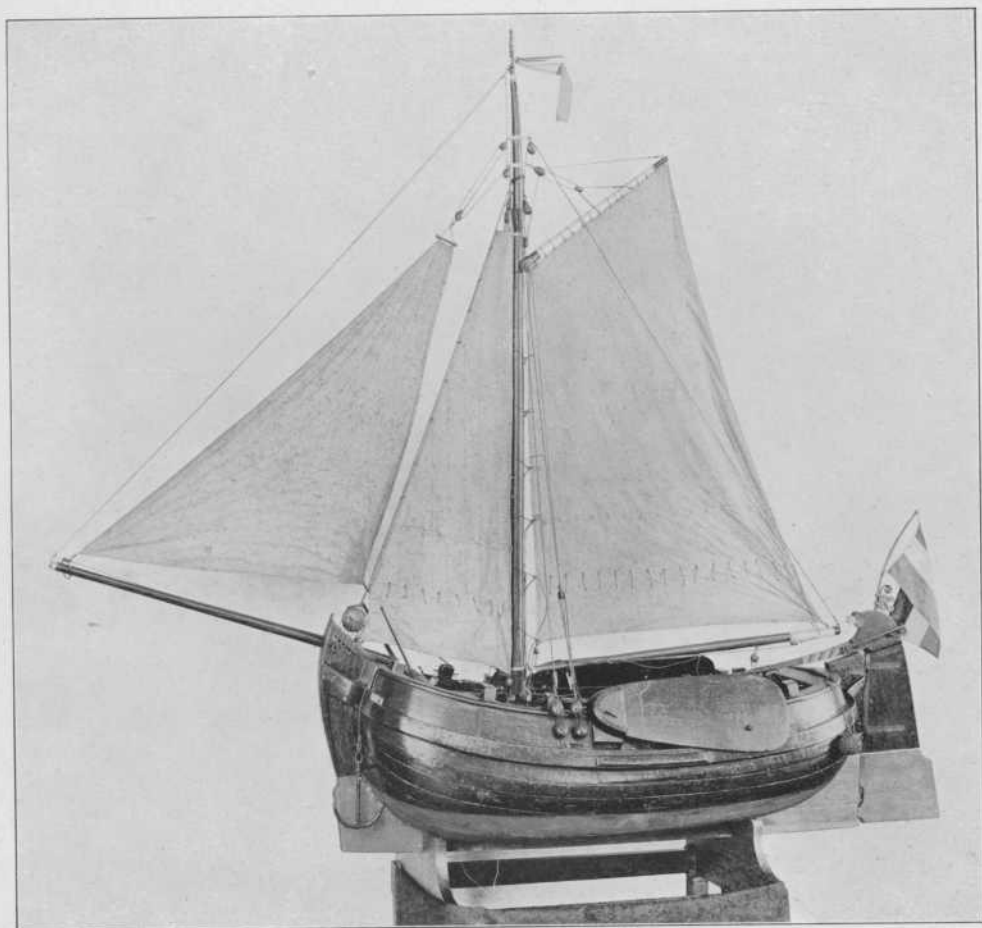
BEZAANSCHUIT VAN PERNIS MIDDEN 19e EEUW
