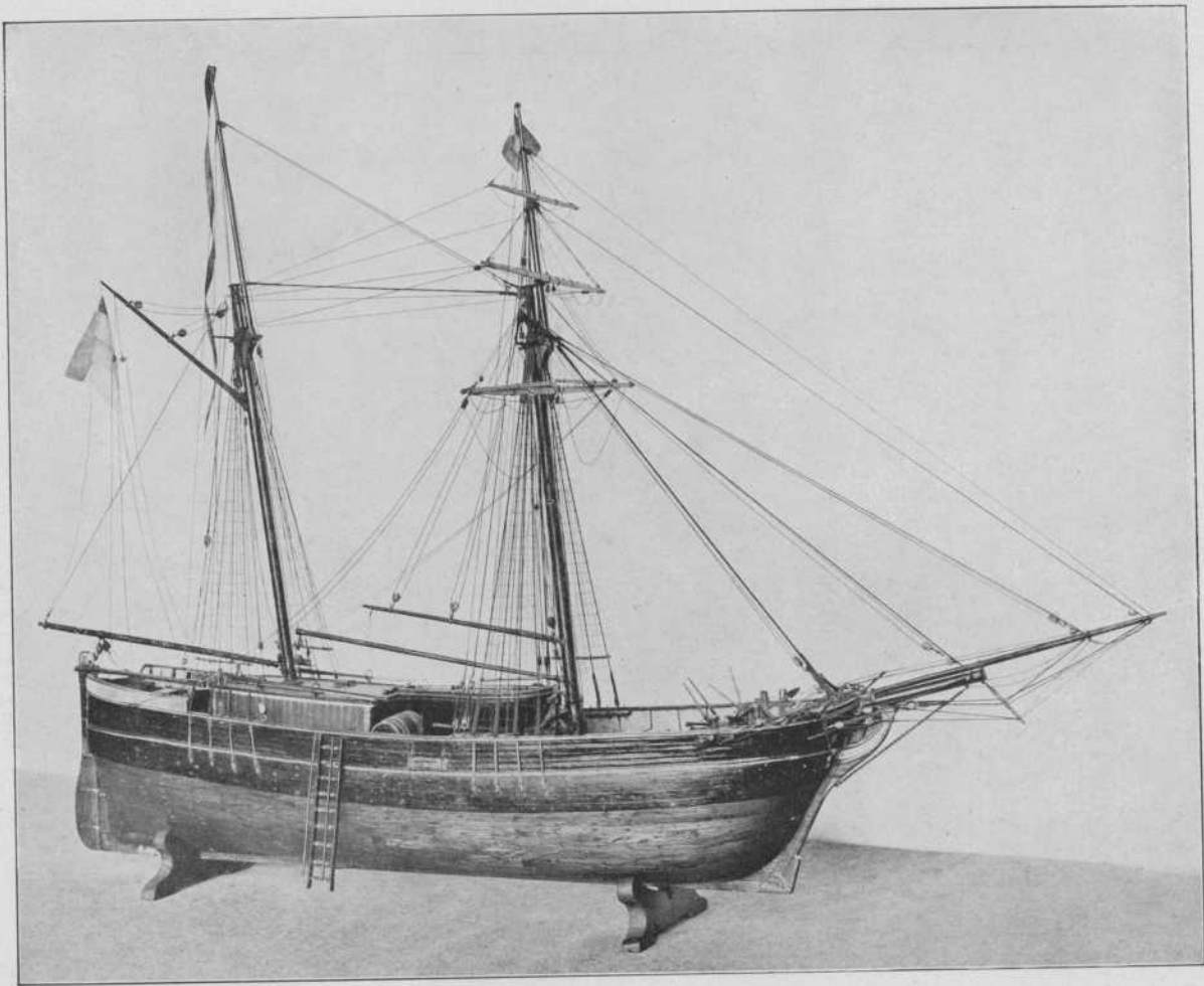
GRONINGER GALJOOT MIDDEN 19 e EEUW
