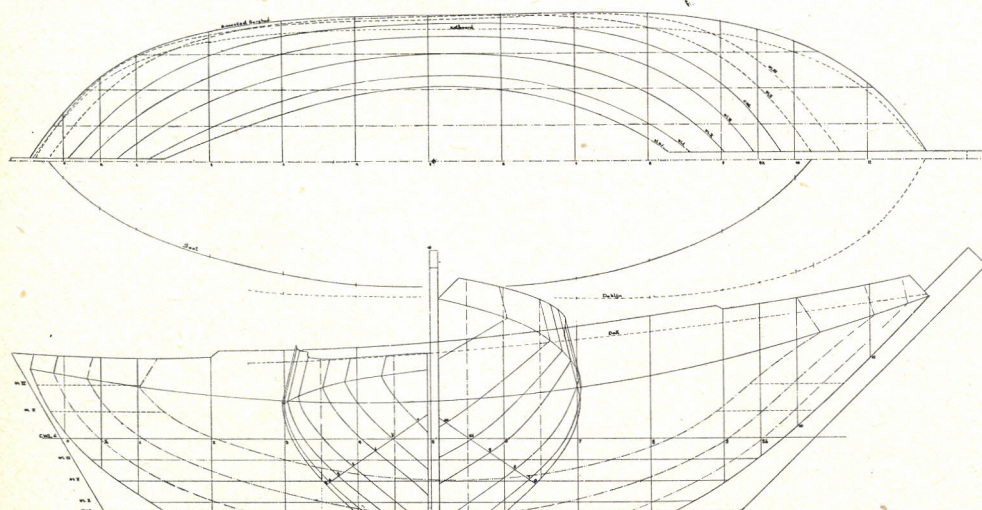
„Schokland”, schokkerjacht, ontwerp Jan van Ommen. Zeiltekening schaal 1 : 120, lijnentekening schaal 1 : 70. Lengte over alles 9 m, lengte waterlijn 7 m, breedte 2.86 m, diepgang 0.70 m, waterver plaatsing 6.30 m 3 . Zeilopperv vlak 41.47 m 2 , grootzeil 27.22 m 2 , botterfok 14.25 m 2 , stag fok 6.12 m 2 .
