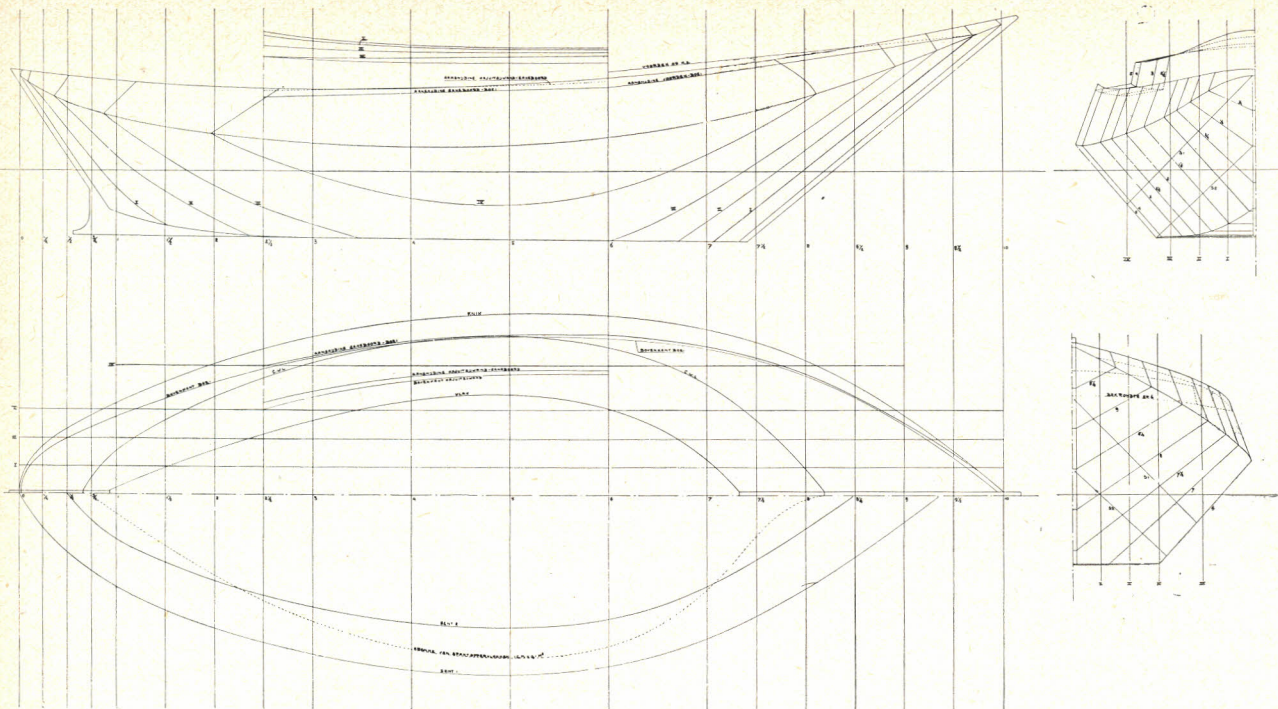
„Zeeland”, h aars jacht, werp J. A. Jon Zeiltekening schaal 1 : lijnentekening schaal 1 : Lengte over a 9.37, lengte wa lijn 7 m, bre 3.36 m, diepg 0.66 m, water plaatsing 6.70 Zeiloppervlak m 2 , grootzeil m 2 , stagfok 8.9 kluiver 6.6 m
