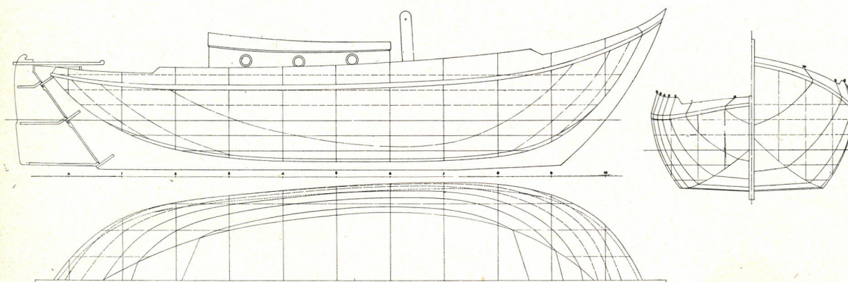
„Kleine Beer”, botte jacht, ontwerp J. v Nek. Zeiltekeni schaal 1 : 120, lijnen kening schaal 1 : Lengte over alles 8.2 lengte waterlijn 7 breedte 2.66 m, die gang 0.65 m, waterve plaatsing 4.90 m 3 . Ze oppervlak 34.8 m 2 , grootzeil 19.8 m 2 , bo terfok 15 m 2 , stagf 8.7 m 2 , kluiver 9 m 2 .
