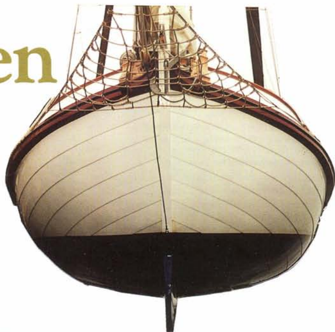
VA 127 Bolle Ontwerp André Hoek Bouw Wilstra, Bolsward, 1995 Eigenaar D. van Dijck Afmeting 12,15 x 4,30 m Gewicht 17,3 ton, 18,1 ton na weging Een relatief grote waterverplaatsing, dat resulteert in een volle spantvorm. Mooi en evenwichtig verloop van de gangen.
