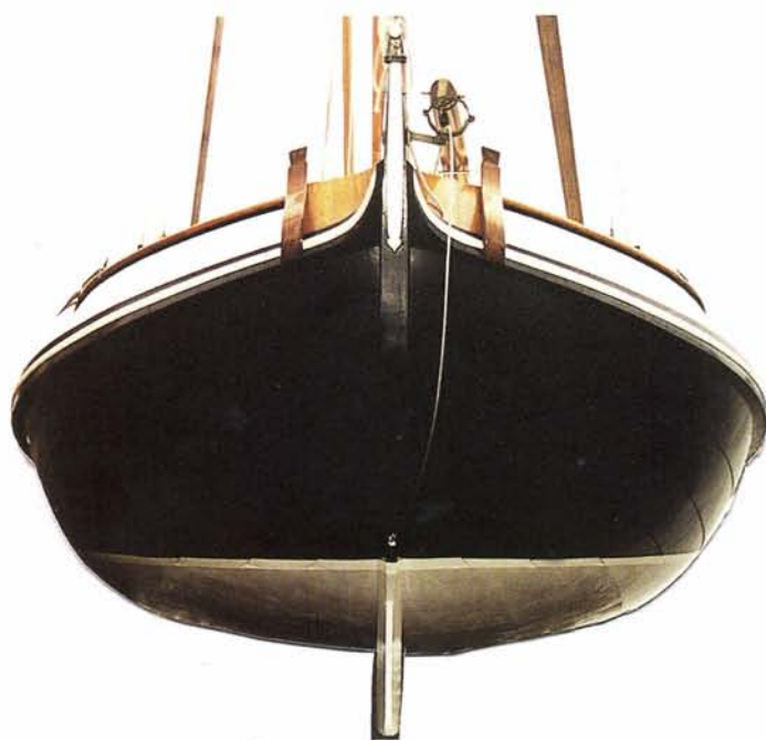
VA 106 Windwaarts Ontwerp ir M. de Groot Bouw Engelaer, 1990 Eigenaar ir. M. de Groot Afmeting 13,60 x 4,50 m Gewicht 18,3 ton, 16,7 ton na weging Er zijn twee aken naar dit model gebouwd en we zien een relatief kleine waterverplaatsing en een weke kim.
