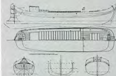
ZUID-HOLLANDSE STATIETJALK
