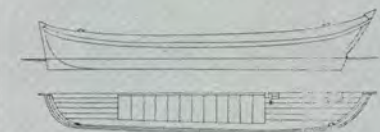
SPITSPRAAM
