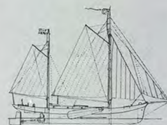
KLIPPER „LEONORA“
