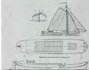
TJALK
