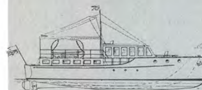
DIESEL-MOTORKRUISER ONTWERP A. TANS
