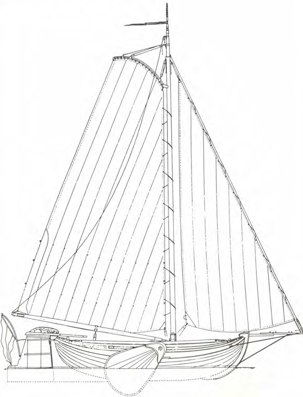
Zeiltekening van de tjotter 'De Vrouwe Anna Beatrijs', grootzeil 17 m 2 , fok 8.25 m 2
