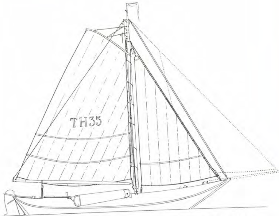
Zeiltekening van de Tholense hoogaars 'TH 35', grootzeil 40.1 m 2 , fok 19.1 m 2 , kluiver 20.2 m 2
