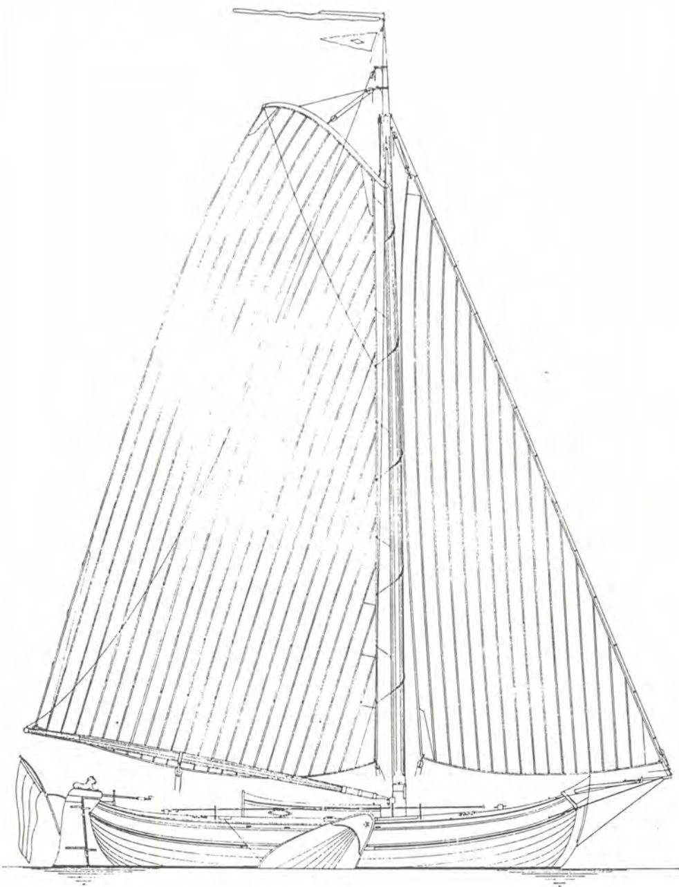
Zeiltekening van de boeier 'Constanter', grootzeil 38.5 m 2 , fok 19.5 m 2
