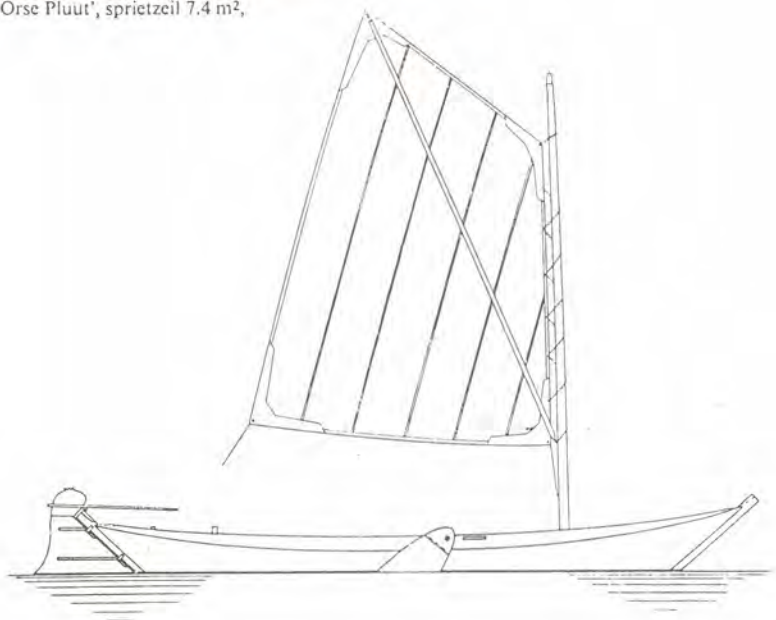
Zeiltekening van de Giethoornse punter 'Orse Pluut', sprietzeil 7.4 m²,
