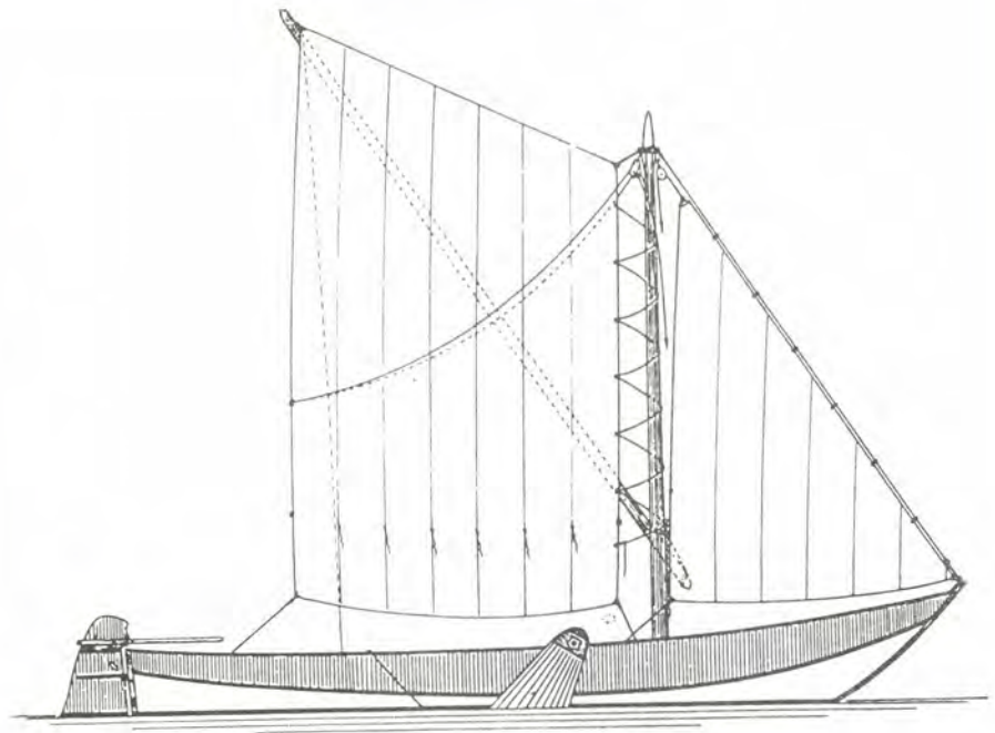
Zeiltekening van een zalmschouw, grootzeil 11.75 m², fok 4.25 m²
